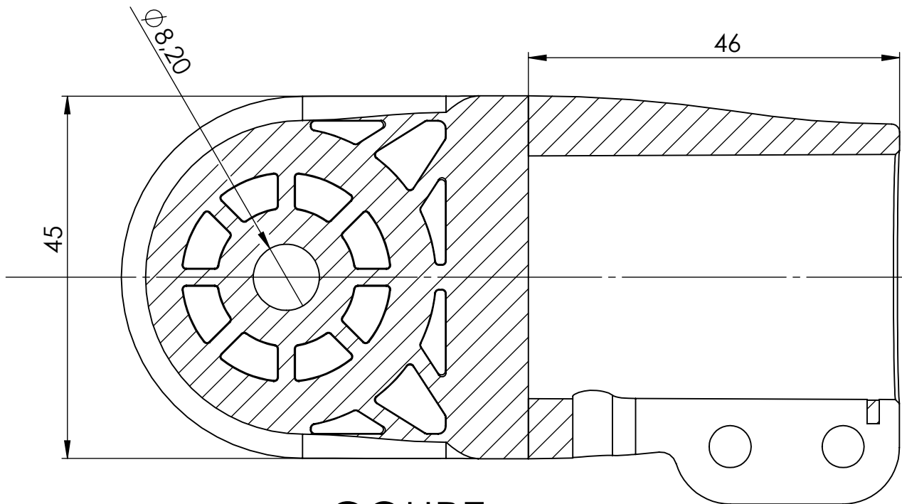
COUPE A-A
